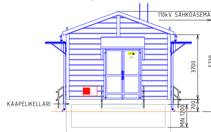
LEIKKAUS A-A, PÄÄVIEN SUUNNASTA KATSOTTUNA
