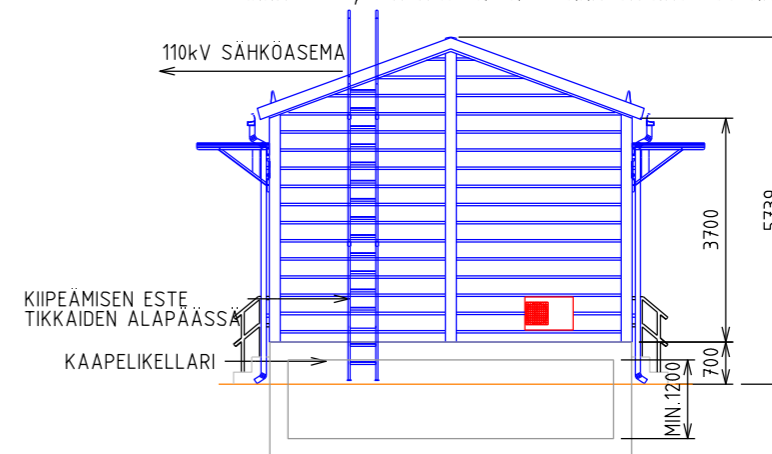
LEIKKAUS C-C, SCADA HUONEEN SUUNNASTA KATSOTTUNA
