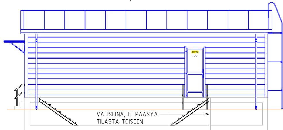
LEIKKAUS B-B, PÄÄMUUNTAJAN SUUNNASTA KATSOTTUNA
