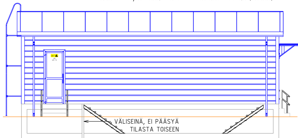
LEIKKAUS D-D, ASEMAN ULKOPUOLELTA KATSOTTUNA (TAKAA)
