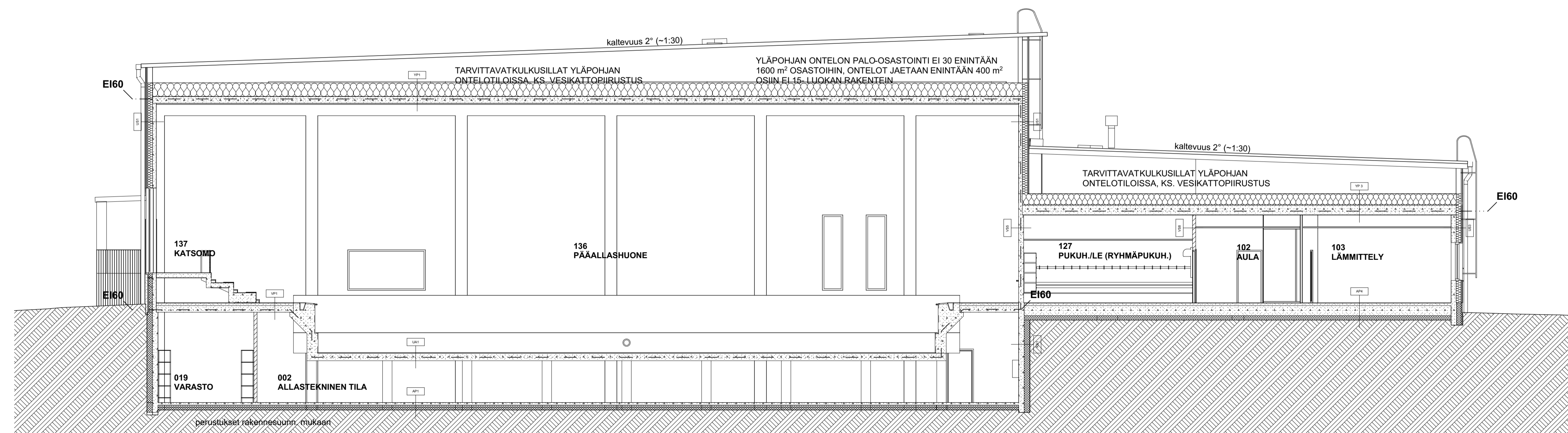
Leikkaus B-B
