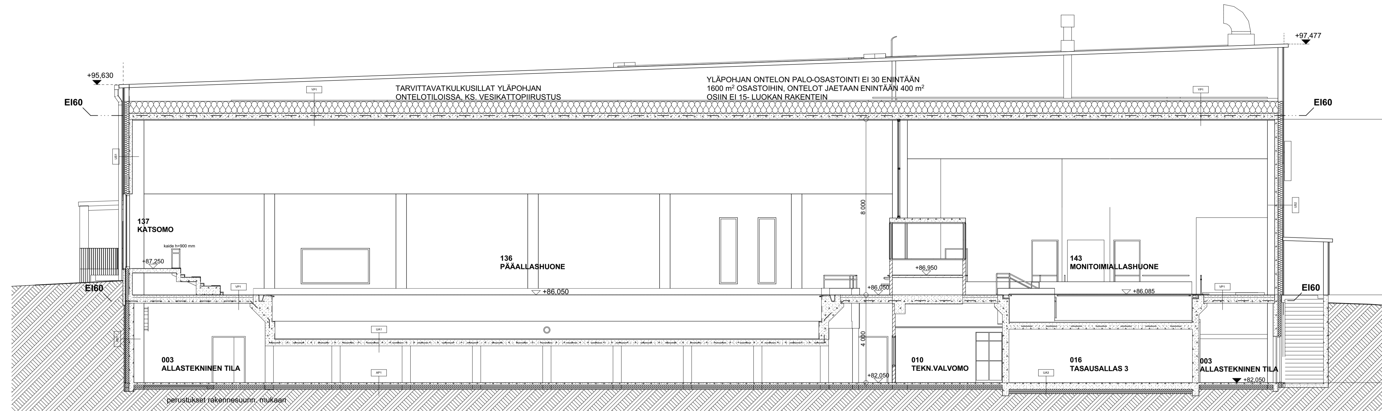
Leikkaus A-A
