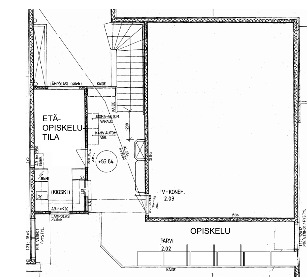
POHJA 2.KRS 1:100
