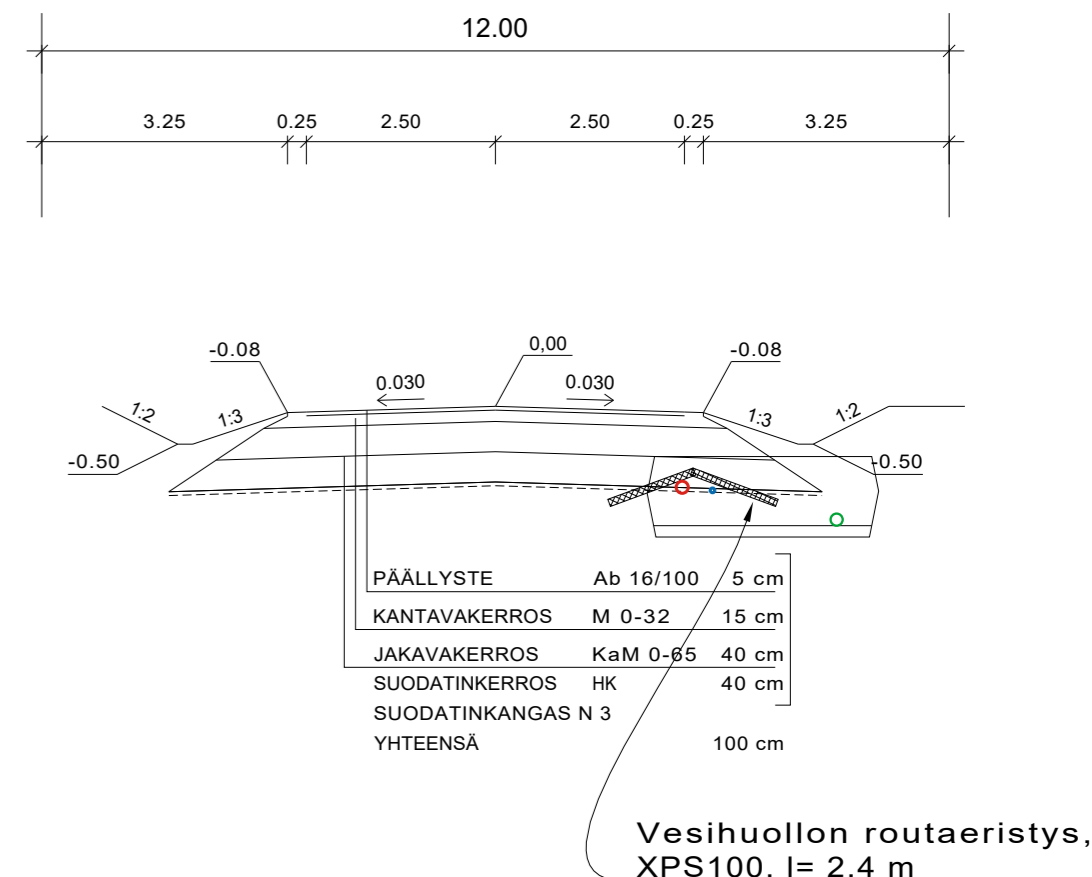
TYYPPIPOIKKILEIKKAUS PAALULTA 280 1:100
